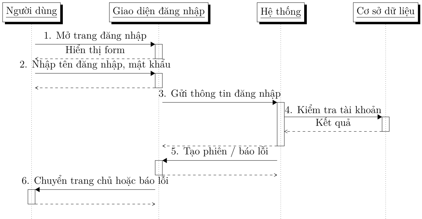
Figure 1: Sequence diagram UC01 – Đăng nhập
